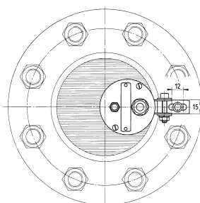
Befestigung «Sch»
